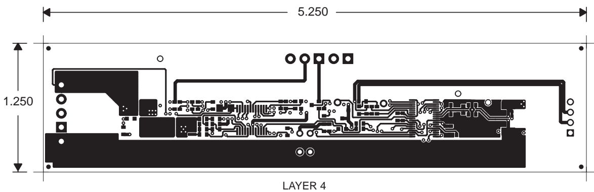
Figure 4-6. Layer 4
